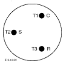
Подсоединение двигателя
