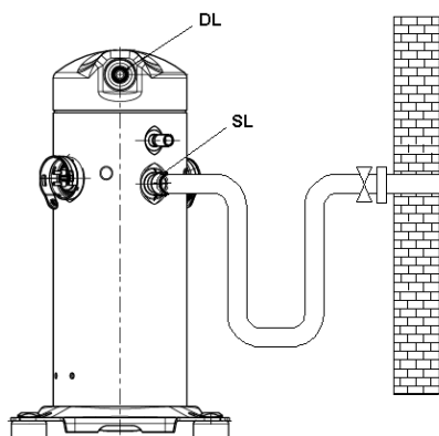
Рис. 7: Конструкция трубопровода
